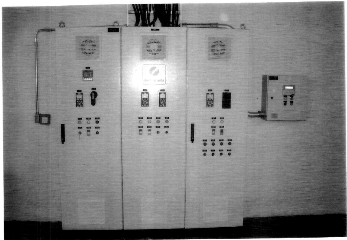
PAINEL ELÉTRICO CENTRAL DE AR.
