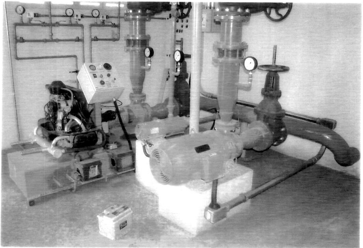
BOMBAS LINHA DE HIDRANTE.
