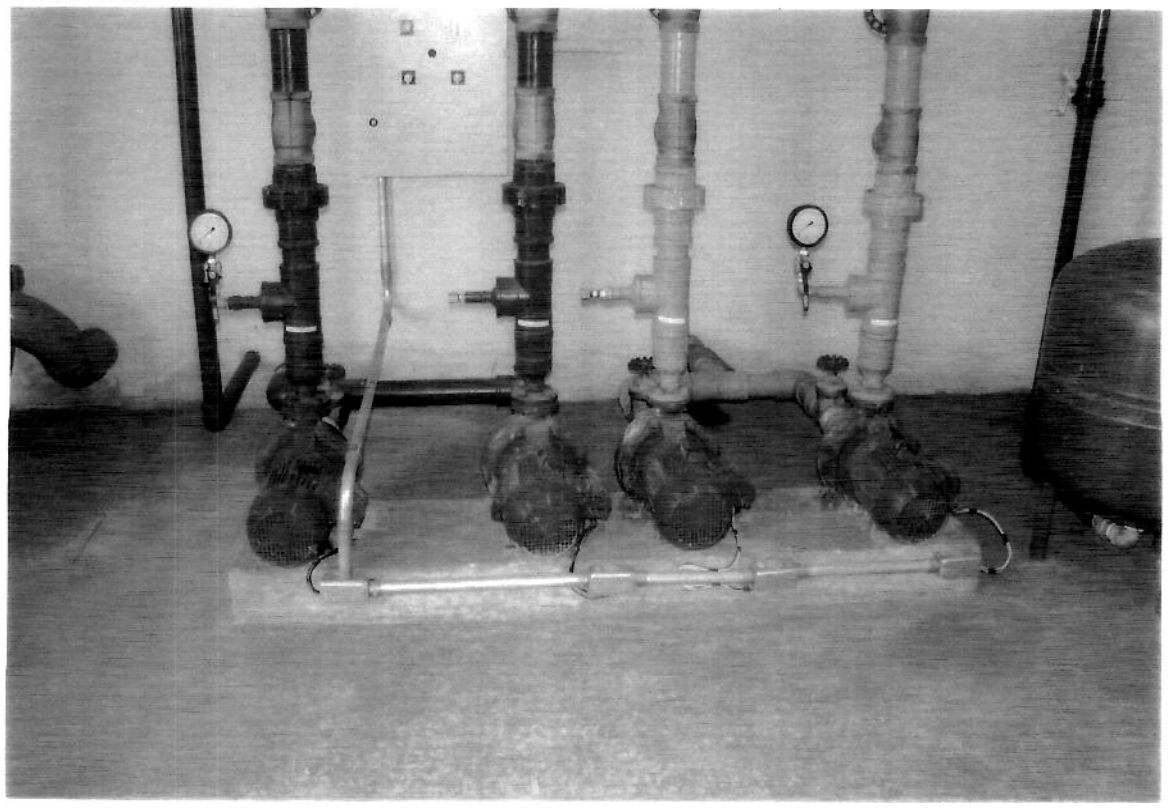
BOMBAS D'ÁGUA.
