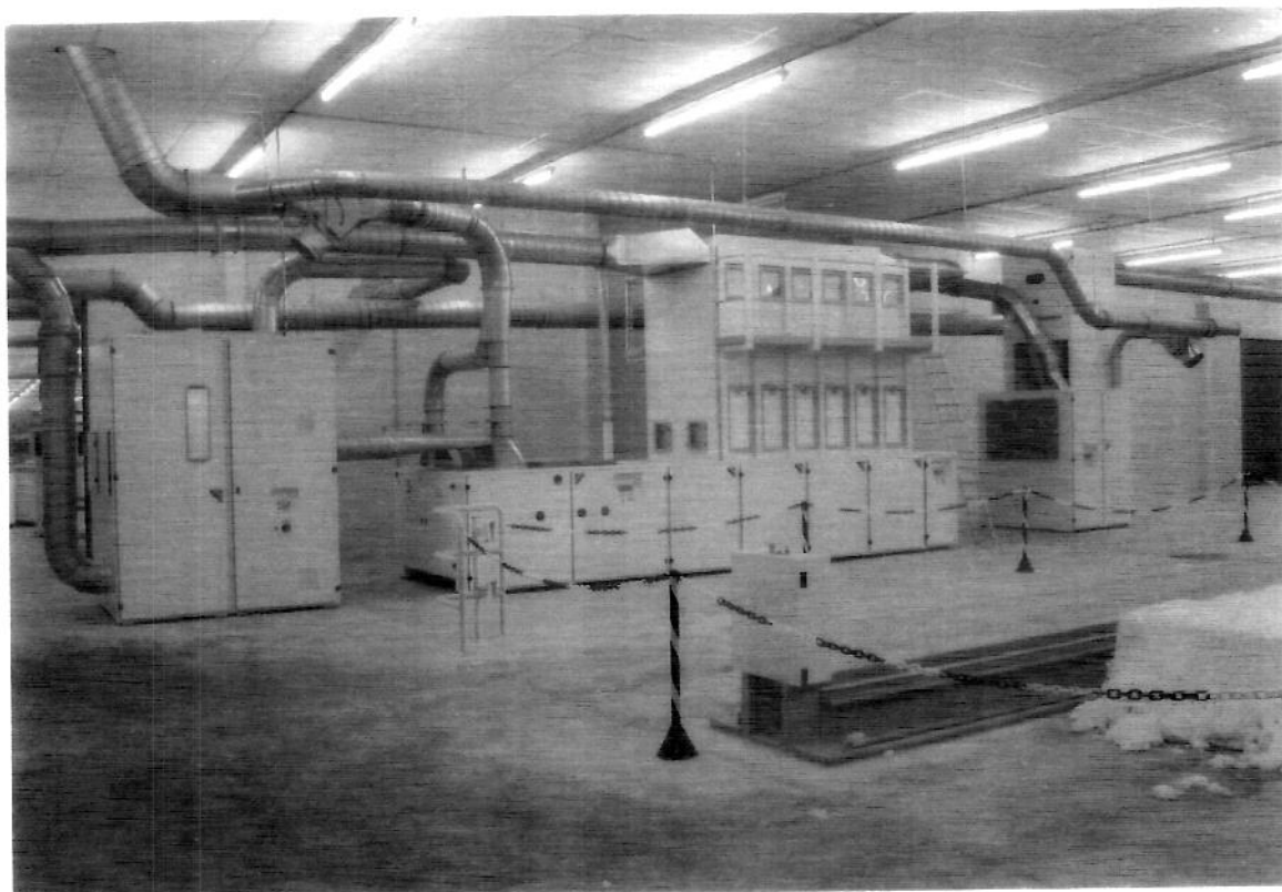
LINHA DE ABERTURA.
